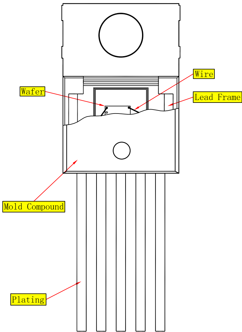
正视图
