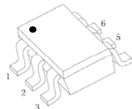
SOT-23-6L
